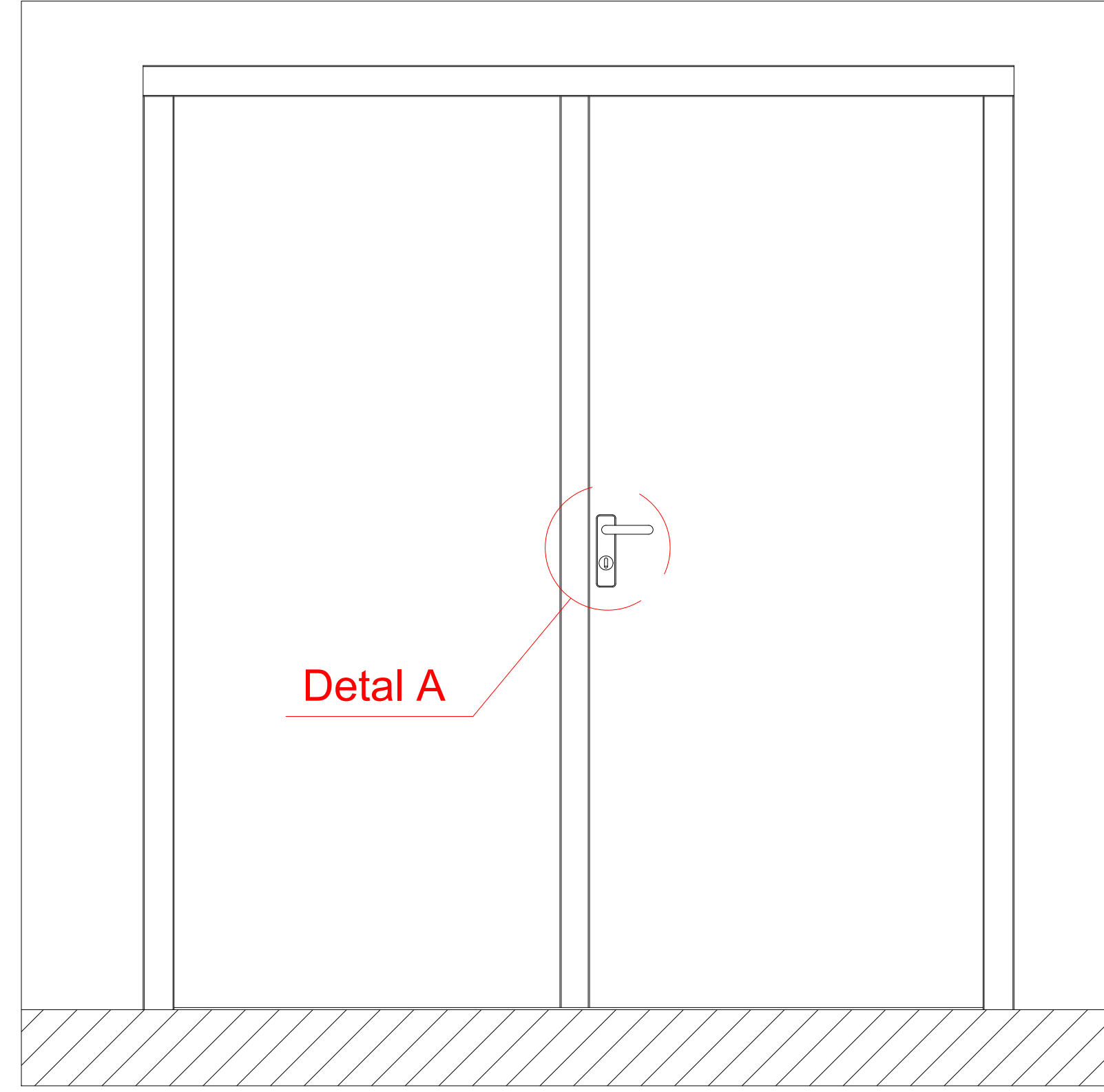
2 İç görünüşü
